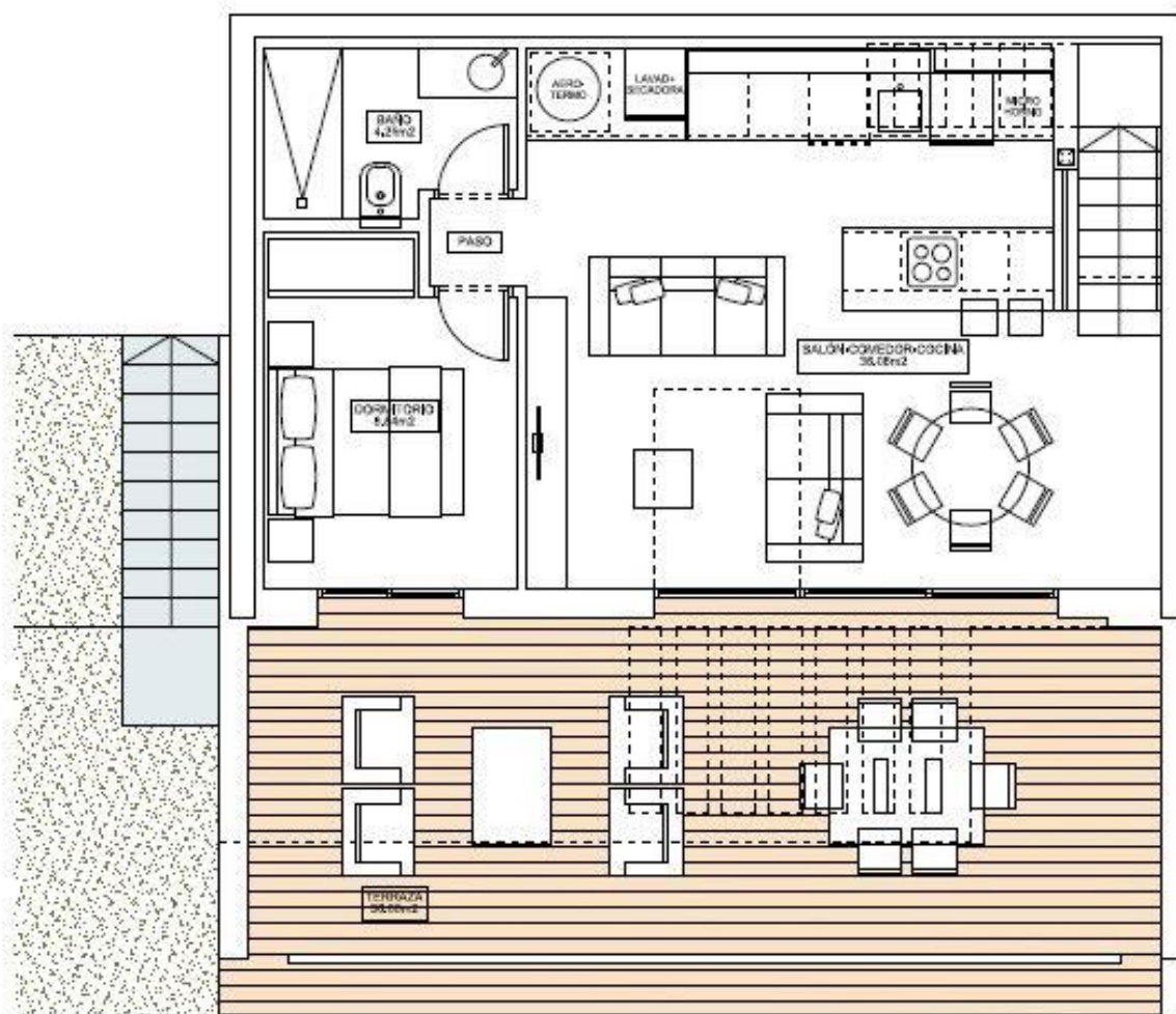
PLANTA PRIMERA
