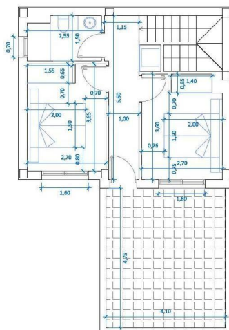
PLANTA PRIMERA
